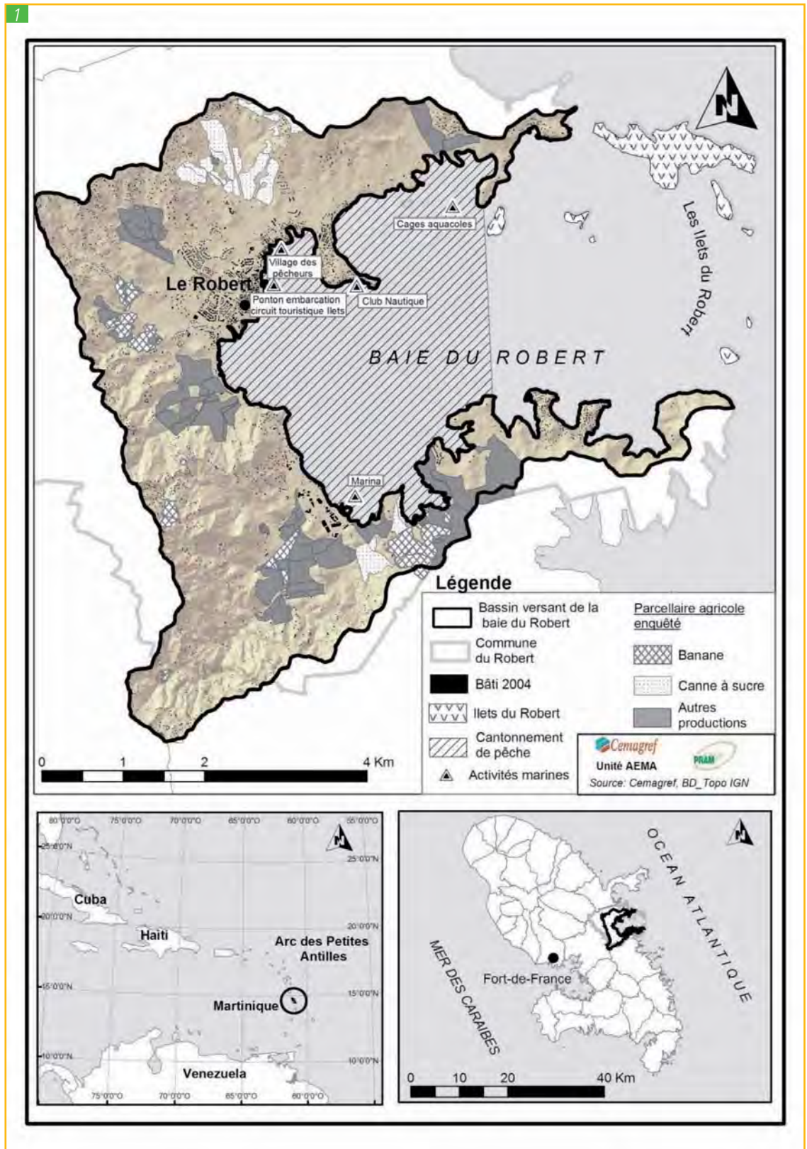
Figure 1 : présentation du bassin versant de la baie du Robert (Pinte, 2007).
