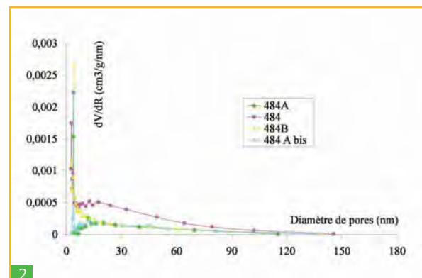
Figure 2 : distribution en taille des pores des échantillons de sols 484 ( 5,9 % allophane) bruts et amendés avec les deux composts 484A ( 484A bis) et 484B.
